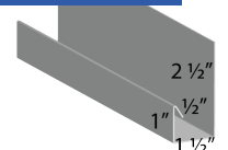
HP Jamb
