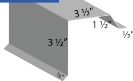
Rake HP
