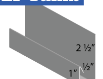
LP Jamb
