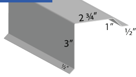
Rake LP
